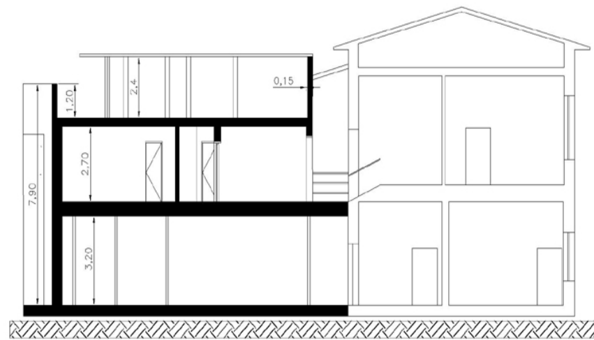
Sezione trasversale
