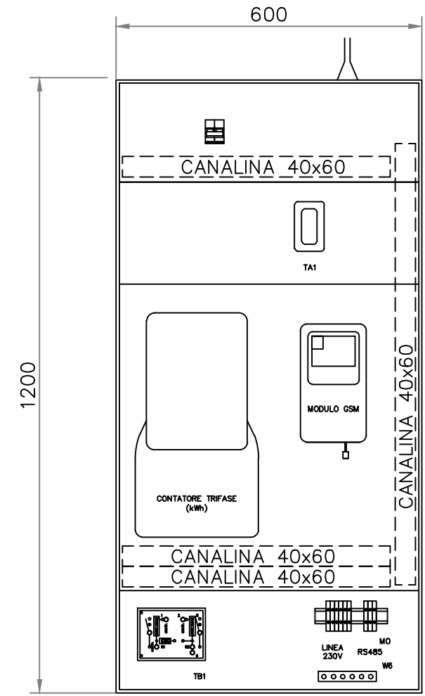
PIASTRA INTERNA
